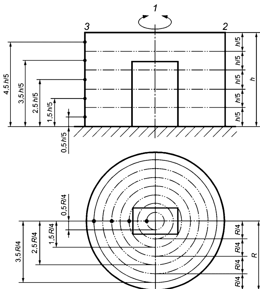
1 - ось вращения микрофонов при сканировании; 2 - размеры соответствующих площадей частей поверхности цилиндра; 3 - положения траекторий сканирования микрофонов; h - высота цилиндра; R - радиус цилиндра
