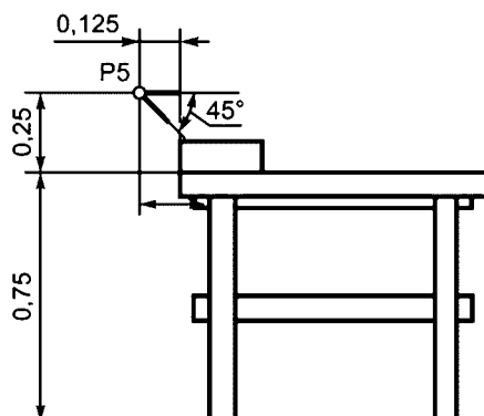
d) Оператор в положении сидя для настольного оборудования (при отсутствии клавиатуры)
