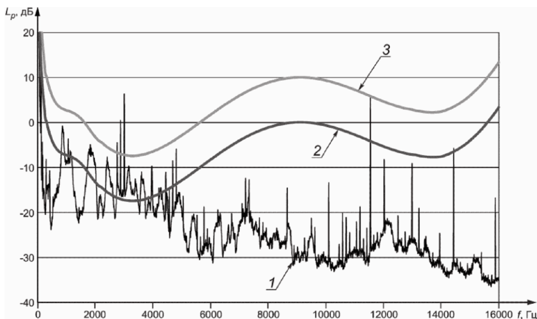
1 - БПФ-спектр; 2 - P_1(f) ; 3 - P_1(f) + 10 дБ; f - частота; L_p - уровень звукового давления (относительно 20 мкПа)
