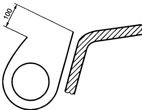
Рисунок ДА.1 - Заправка листа бумаги
