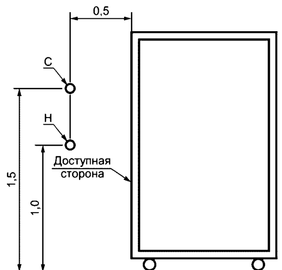
Рисунок ДА.6 - Рабочие места оператора в положениях "стоя" (С) и "нагнувшись" (Н) для стоечных систем
