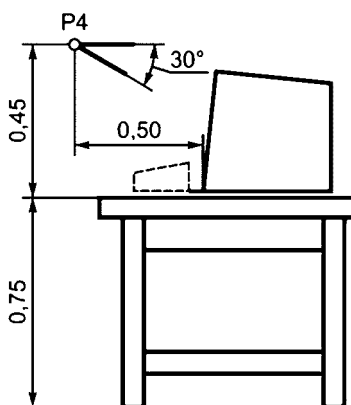
d) Оператор в положении сидя для настольного оборудования (при отсутствии клавиатуры)
