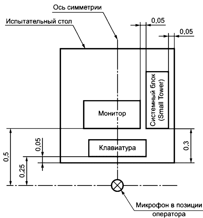
Рисунок ДА.4b - Установка настольного оборудования с системным блоком типа "Small Tower"
