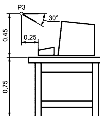
c) Оператор в положении сидя для настольного оборудования (при наличии клавиатуры)
