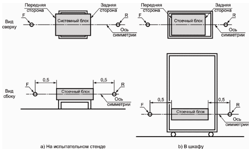
Рисунок ДА.5 - Переднее (F) и заднее (R) расположение оператора для стоечных блоков
