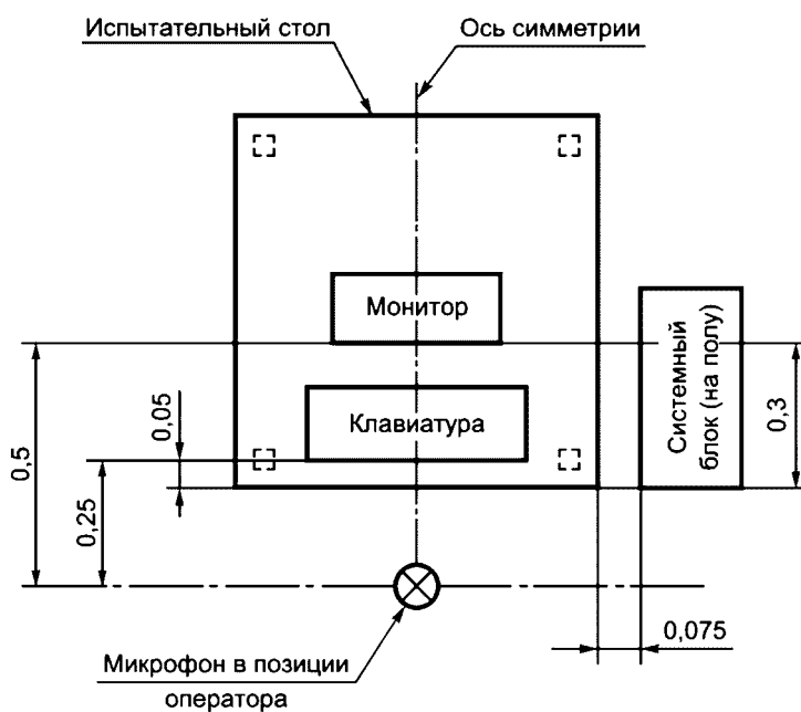
Рисунок ДА.4с - Установка оборудования, имеющего настольные
